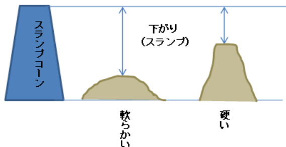
コンクリートの硬さによるスランプの違い
