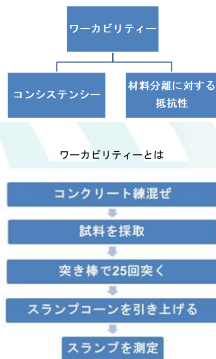
スランプ試験の手順
