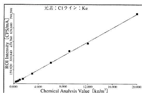
検量線の例 (アワズテック社技術資料より)
