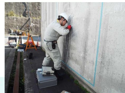
ひび割れ深さ測定の例
