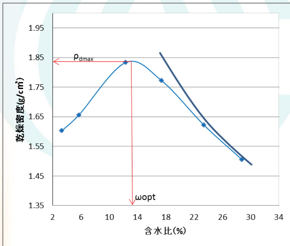
締固め曲線
