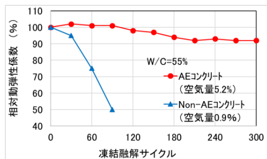
相対動弾性係数の変化例
