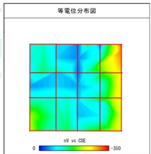
図-2. 自然電位測定結果例
