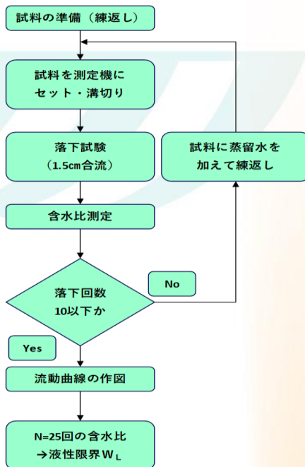
試験フロー図 (液性限界試験)
