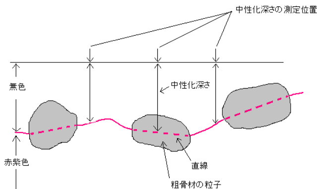
図-1 測定箇所粗骨材の粒子がある場合の測定例
